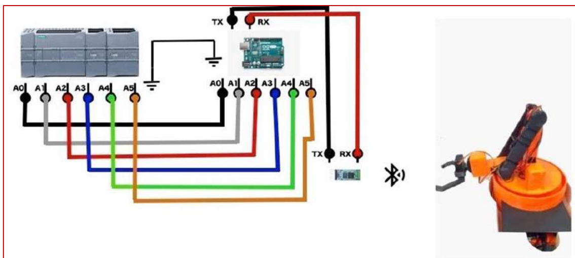
Figura 9. Integração CLP-Arduino
