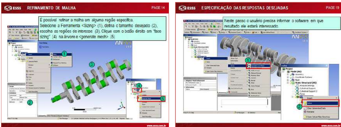
Figura 2 – Detalhe do tutorial passo a passo para o 1º exercício de Análise Estática Linear de um Virabrequim, refinamento da malha e pós-processamento de resultados.
