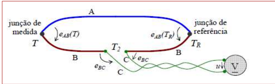
Figura 2- Circuito do Termopar
